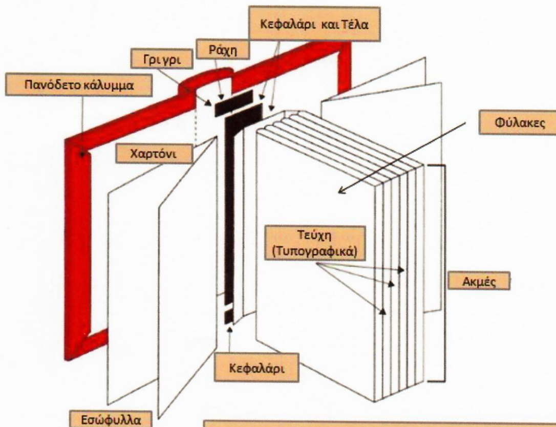
Σχεδιάγραμμα πανόδετης βιβλιοδεσίας
